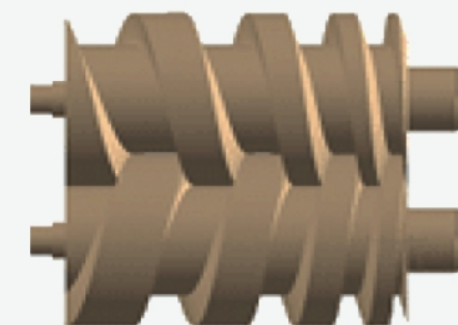
变螺距螺杆
