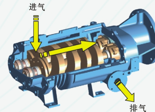
干式螺杆真空泵的工作原理图
